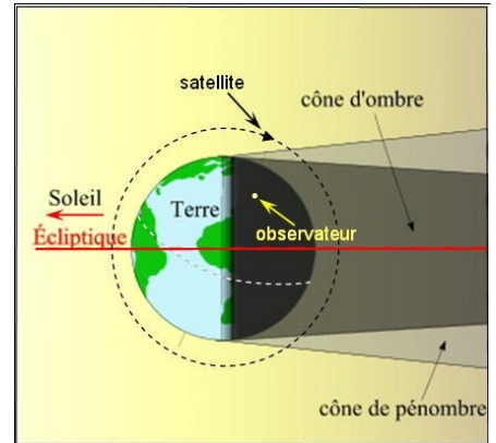
Illustration 2: Schéma de la trajectoire d'un satellite.
