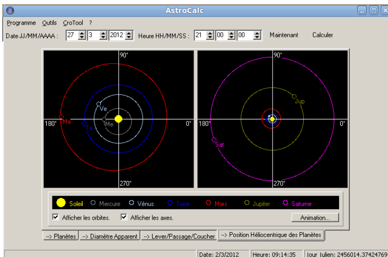
Illustration 5: Copie d'écran du logiciel AstroCalc.
