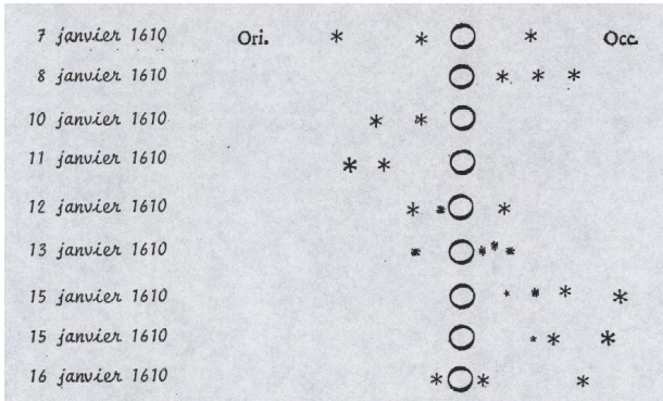
Illustration 7: Relevé des observations de Galilée sur les satellites de Jupiter.
