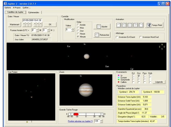
Illustration 6: Copie d'écran du logiciel Jupiter2.
